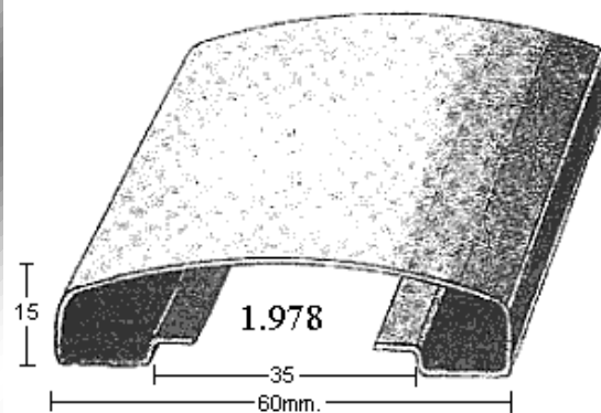
PASAMANOS 1978 (1 ó 1,2mm.)
