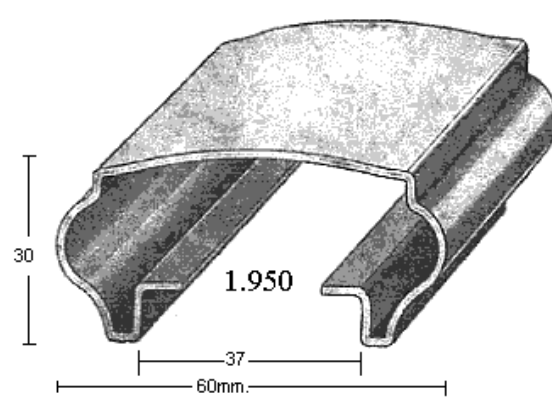
PASAMANOS 1950 (1 ó 1,5mm.)
