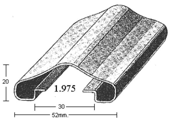
PASAMANOS 1975 (1 ó 1,5mm.)
