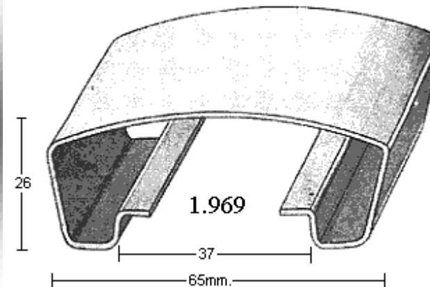
PASAMANOS 1969 (1 ó 1,5mm.)
