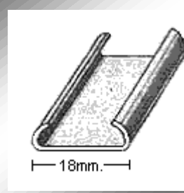
PERFIL 1217 (0,8mm.)
