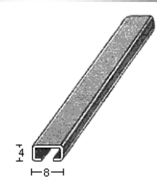
PERFIL 2441 (0,8mm.)
