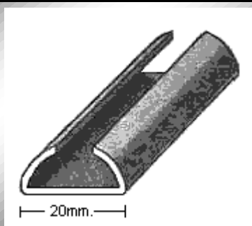
PERFIL 1808 (1mm.)
