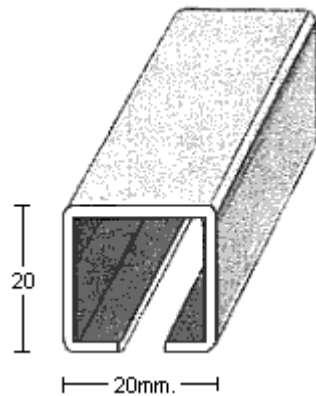
PERFIL 2402 (2mm.)
