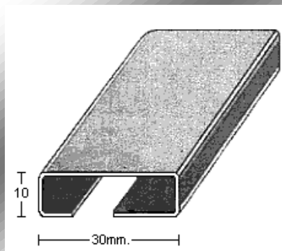
PERFIL 2394 (1mm.)
