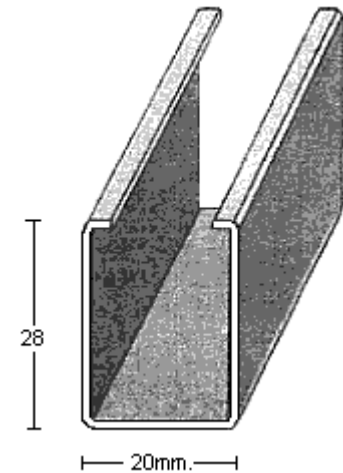
PERFIL 2483 (1mm.)
