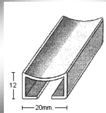
PERFIL 2479 (1,5mm.)
