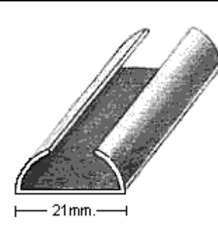
PERFIL 1499 (1mm.)
