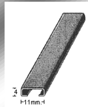
PERFIL 2421 (0,8mm.)
