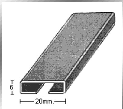
PERFIL 2435 (1,2mm.)
