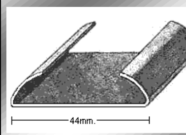
PERFIL 1285 (1,2mm.)
