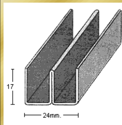
PERFIL 2445
