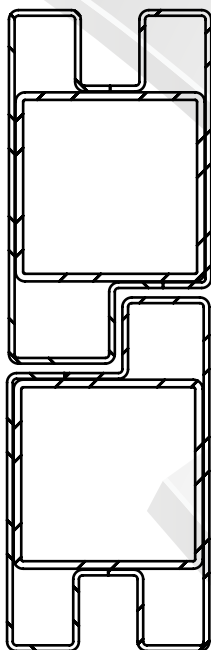
SECCIÓN B-B 90,00° ESCALA 1 : 2
