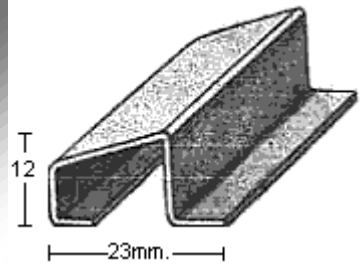
PERFIL 2177 (1mm.)
