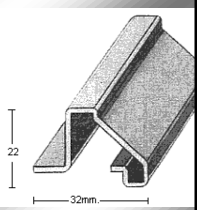
PERFIL 2368 (1,5mm.)
