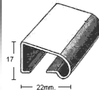
PERFIL 1838 (1mm.)
