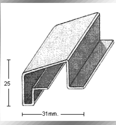
PERFIL 2426 (1,2mm.)
