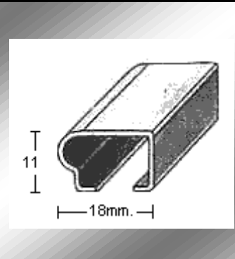
PERFIL 1919 (1mm.)
