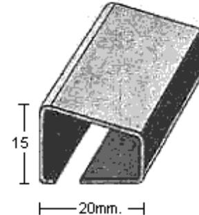
PERFIL 1945 (1mm.)
