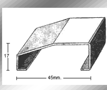
PERFIL 1842 (1,2mm.)
