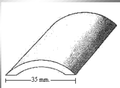
PERFIL 1129=35x3mm.
