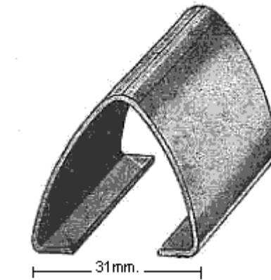
PERFIL 1192
