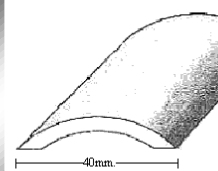
PERFIL 1129=40x3mm.
