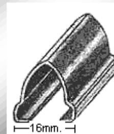
PERFIL 1423
