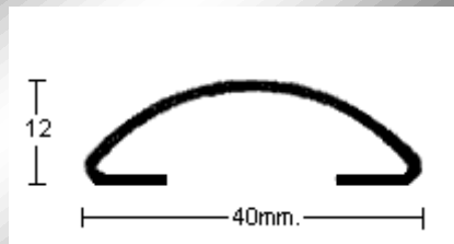
PERFIL 2757
