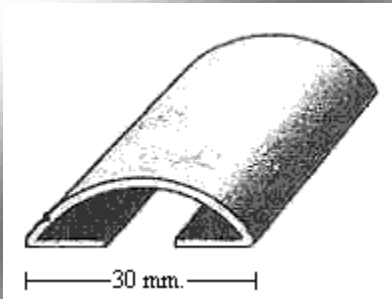
PERFIL 1127=30x1mm.
