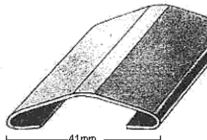
PERFIL 1174
