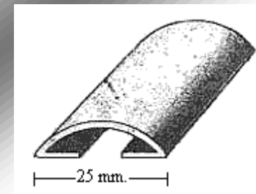
PERFIL 1127=25x1mm.
