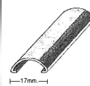
PERFIL 1169
