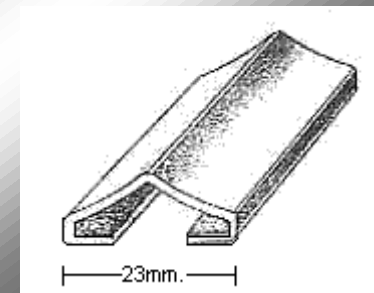
PERFIL 1137
