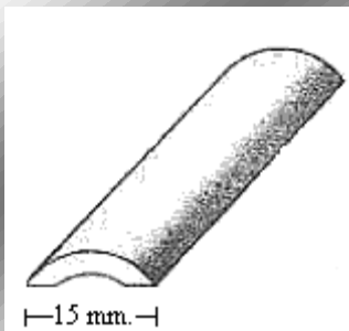
PERFIL 1129=15x1,5mm.
