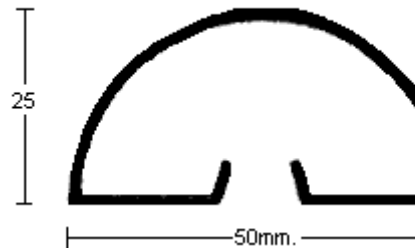
PERFIL 2704
