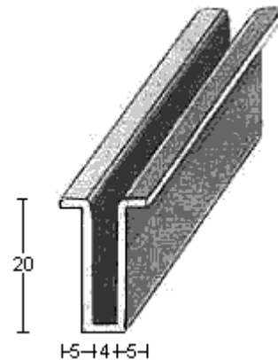
PERFIL 1578 (1,5mm.)
