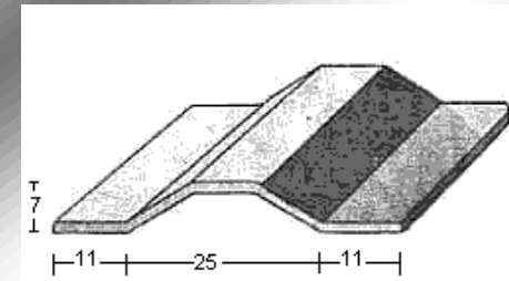
PERFIL 1366 (1,5mm.)
