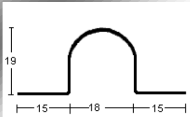
PERFIL 1790 (1mm.)
