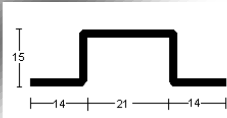
PERFIL 2711 (2mm.)
