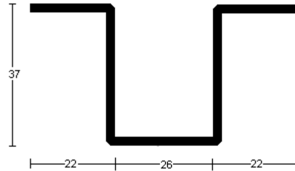
PERFIL 2742 (2mm.)
