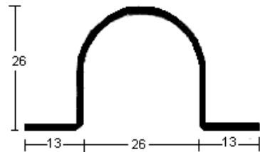
PERFIL 2725 (1,5mm.)
