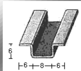
PERFIL 1374 (1mm.)
