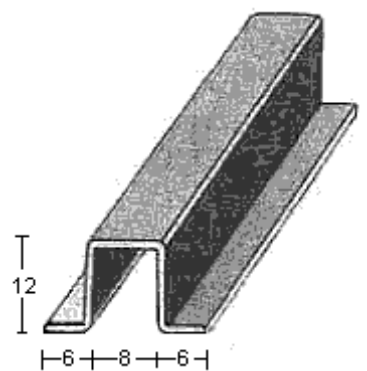
PERFIL 1518 (1mm.)
