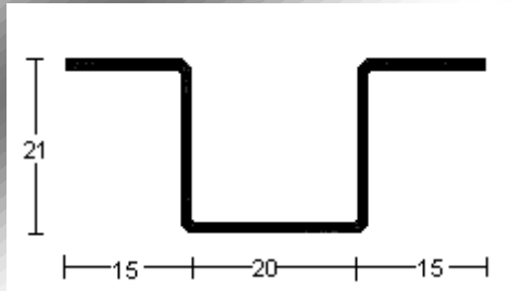
PERFIL 2729 (1,2mm.)
