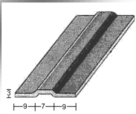
PERFIL 1513 (2mm.)
