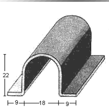
PERFIL 1521 (1,5mm.)
