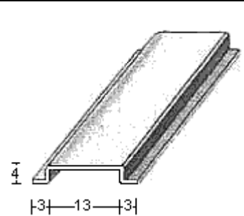
PERFIL 1494 (1mm.)
