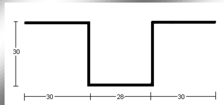
PERFIL 2658 (1mm.)
