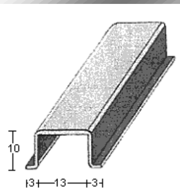
PERFIL 2374 (1mm.)
