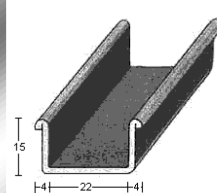
PERFIL 1607 (2mm.)
