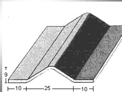
PERFIL 1587 (1,5mm.)
