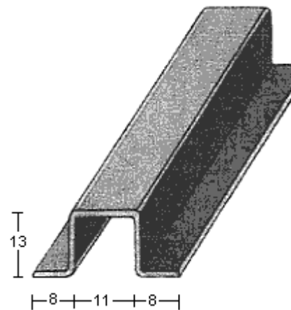
PERFIL 2380 (1,5mm.)
