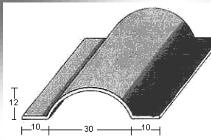
PERFIL 1615 (1,2mm.)
