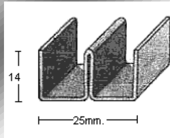
PERFIL 2235
