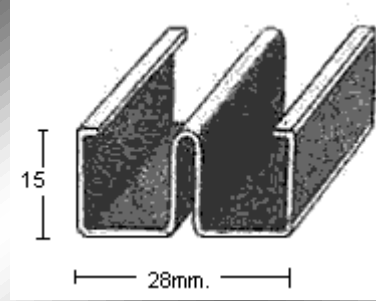
PERFIL 2100
