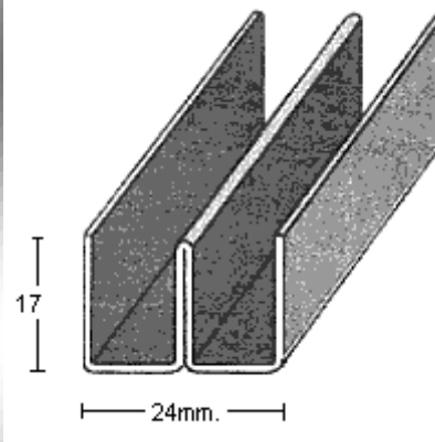
PERFIL 2445
