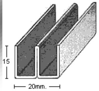
PERFIL 1803
