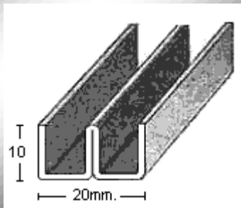
PERFIL 1802
