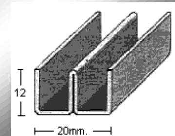
PERFIL 2285
