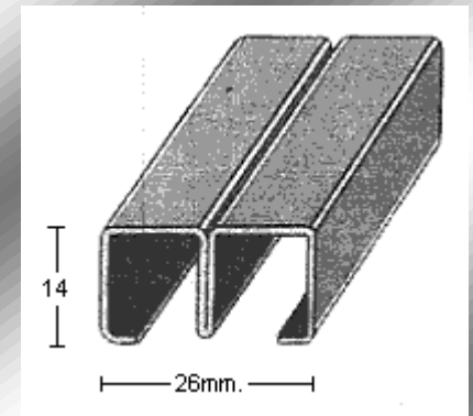
PERFIL 2446
