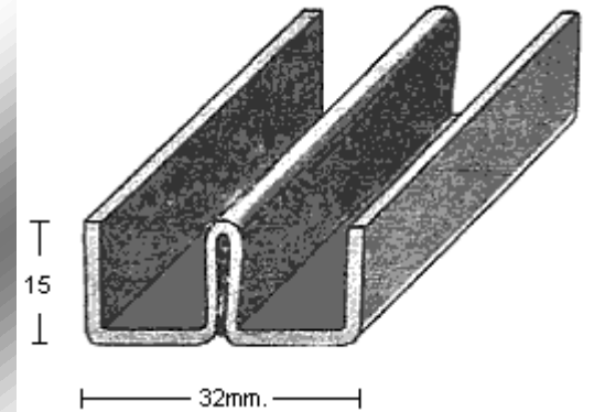
PERFIL 2331
