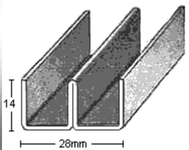
PERFIL 1804
