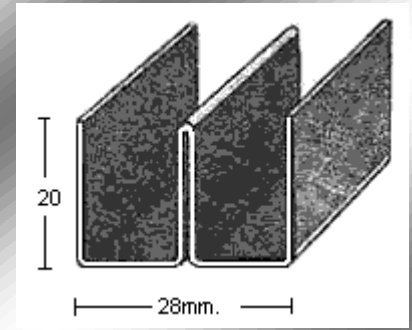
PERFIL 2118
