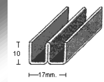
PERFIL 2286
