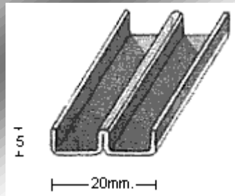
PERFIL 2425
