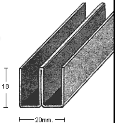
PERFIL 2361
