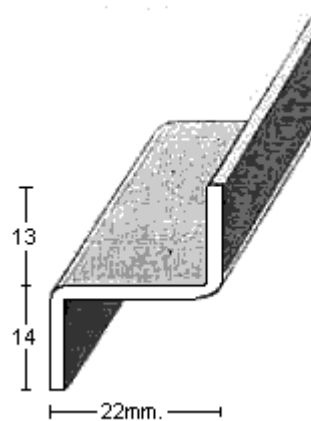
PERFIL 1574 (2mm.)
