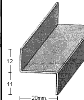
PERFIL 1505 (1mm.)
