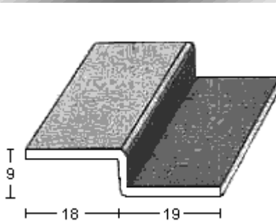
PERFIL 1346 (1,5mm.)
