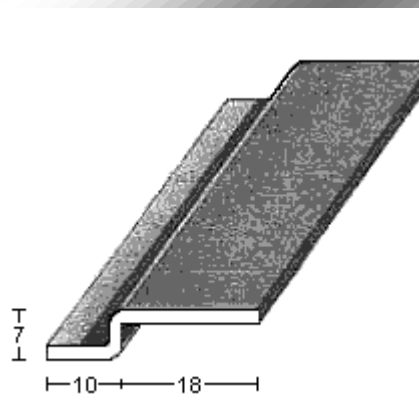
PERFIL 1551 (2mm.)
