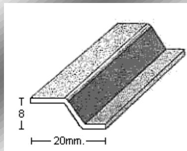
PERFIL 1346 (1,5mm.)
