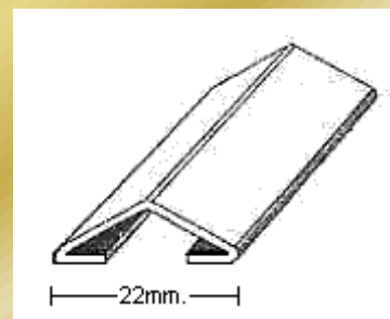
PERFIL 1136
