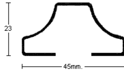
PERFIL 2759
