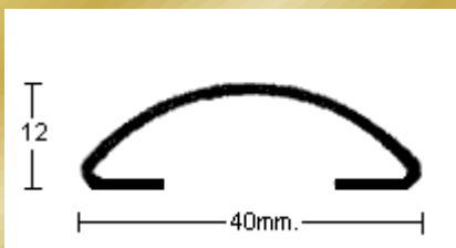
PERFIL 2757
