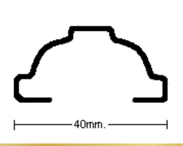
PERFIL 2800
