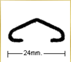
PERFIL 1765
