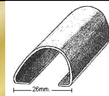
PERFIL 1166
