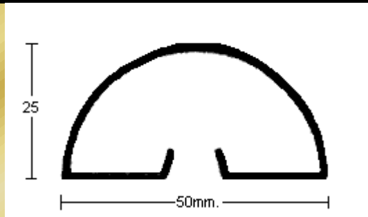
PERFIL 2704
