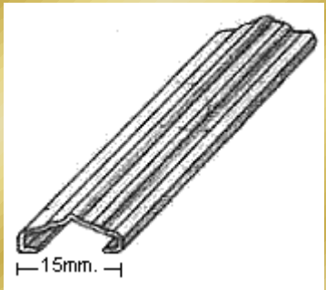
PERFIL 1421
