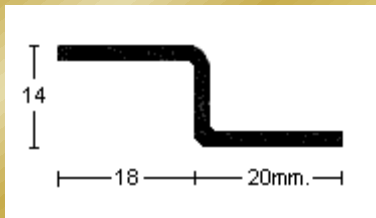
PERFIL 1729 (1,5mm.)
