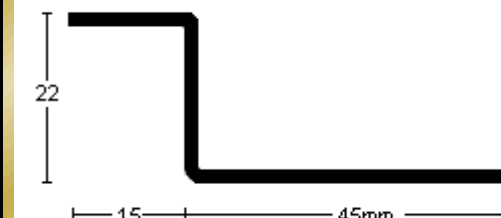
PERFIL 2647 (1,5mm.)
