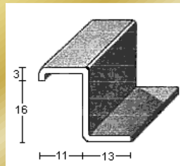
PERFIL 2274 (1,5mm.)
