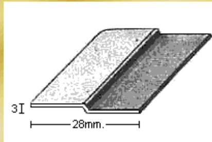
PERFIL 1392 (1mm.)
