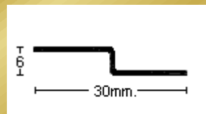
PERFIL 2545 (1mm.)
