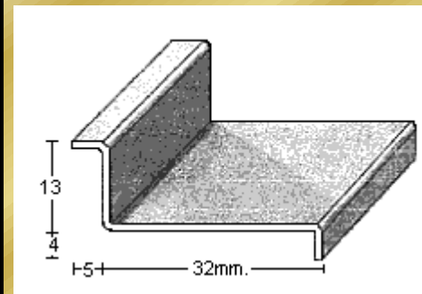
PERFIL 2290 (1,5mm.)
