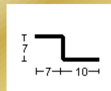
PERFIL 2668 (0,8mm.)
