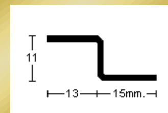
PERFIL 2712 (1,5mm.)
