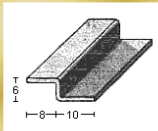
PERFIL 2236 (1mm.)
