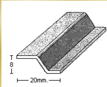
PERFIL 1346 (1,5mm.)
