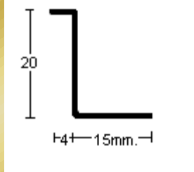
PERFIL 2636 (1mm.)
