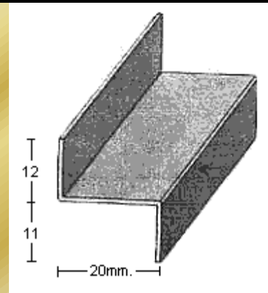
PERFIL 1505 (1mm.)
