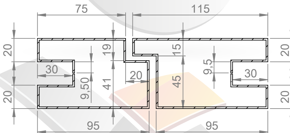
SECCIÓN B-B ESCALA 1 : 2
