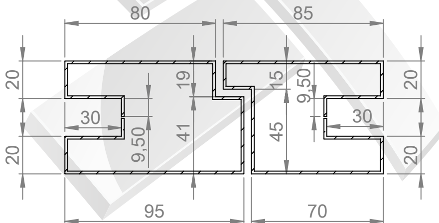
SECCIÓN C-C ESCALA 1 : 2
