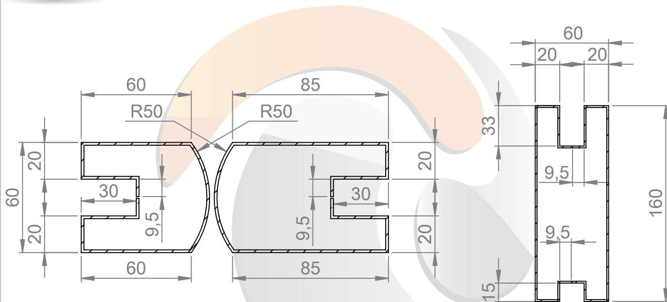
SECCIÓN D-D ESCALA 1 : 2
