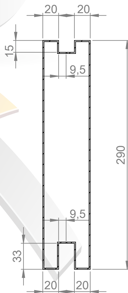
SECCIÓN F-F ESCALA 1 : 3
