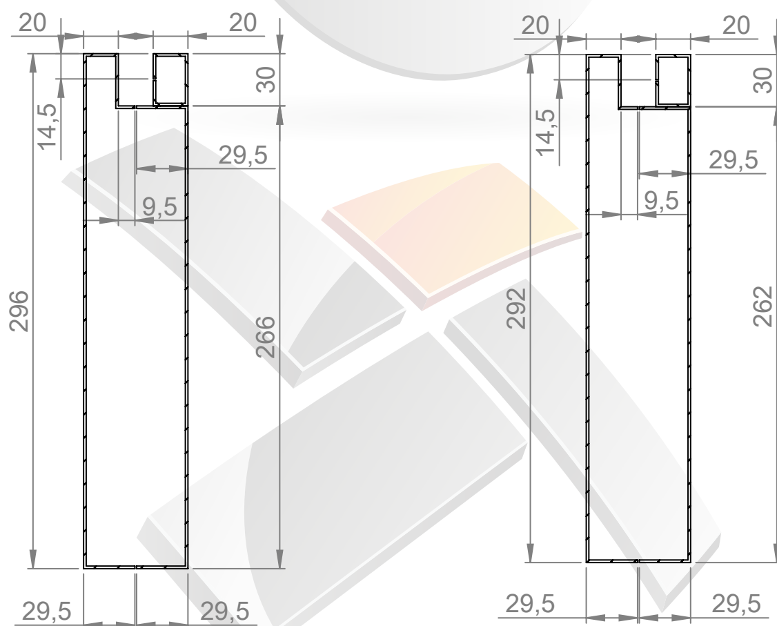
SECCIÓN G-G ESCALA 1 : 3
