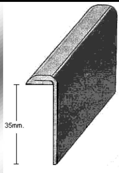
PERFIL 1475 (2mm.)
