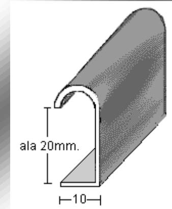
PERFIL 1128 con pestaña=ala 20mm.
