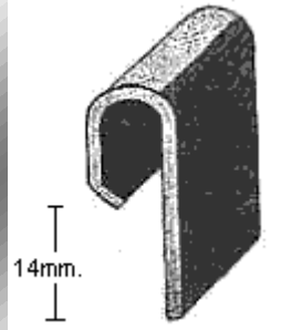
PERFIL 1322 (1,5mm.)
