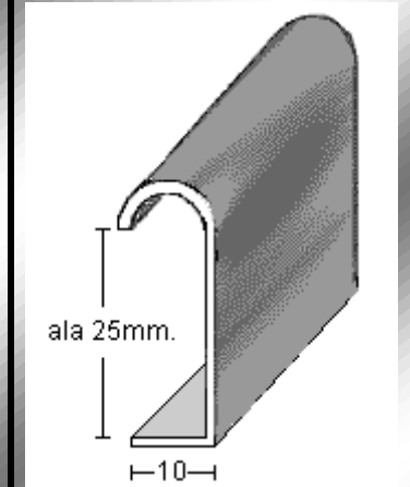
PERFIL 1128 con pestaña=ala 25mm.
