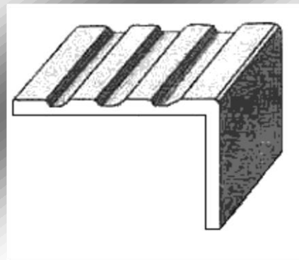
PERFIL 1480=40x23mm. (3mm.)
