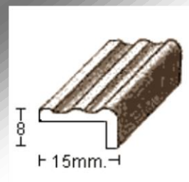
PERFIL 1380=15x15 (2mm.)
