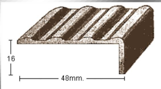
PERFIL 1328 (3mm.)
