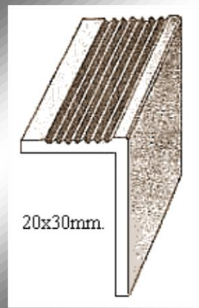
PERFIL 1134=20x30mm. (2mm.)
