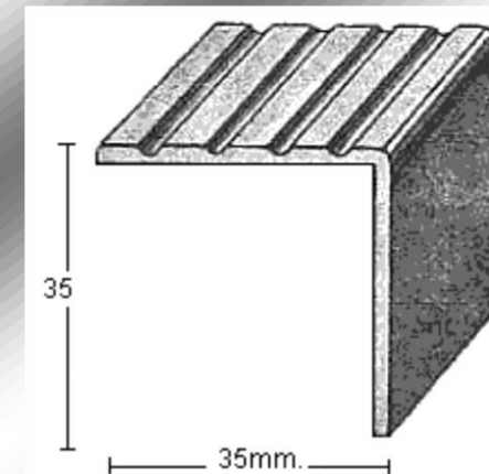
PERFIL 1452 (2mm.)
