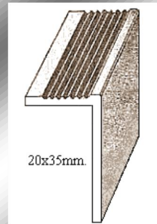
PERFIL 1134=20x35mm. (2mm.)
