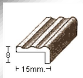
PERFIL 1380=15x8 (2mm.)
