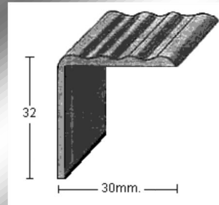
PERFIL 1447 (3mm.)
