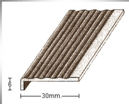
PERFIL 1532 (2mm.)
