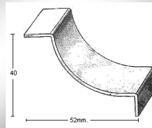
PERFIL 2021 (1mm.)
