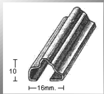
PERFIL 1850 (1mm.)
