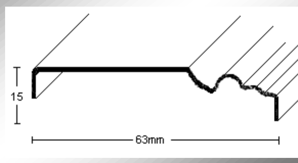
PERFIL 2773 (1,2mm.)
