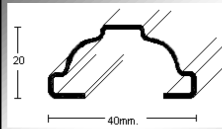
PERFIL 2803 (1,2mm.)
