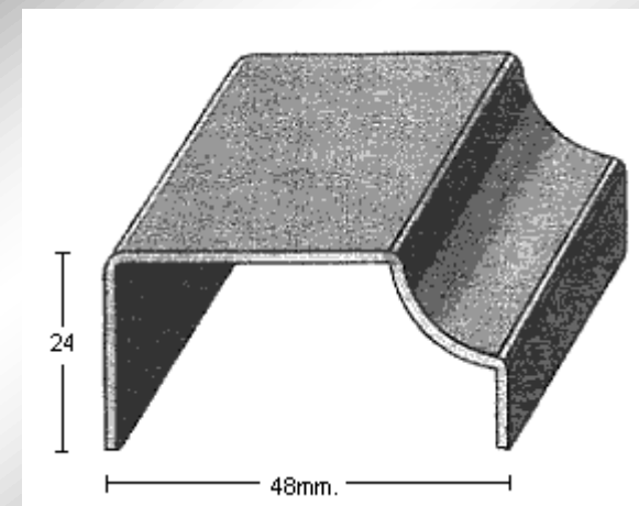
PERFIL 2268 (1mm.)
