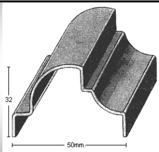
PERFIL 1915 (1,5mm.)
