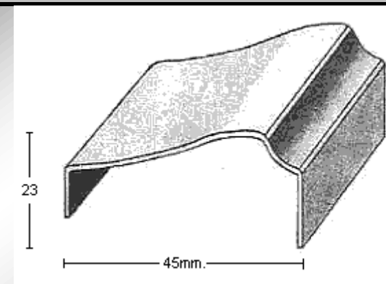
PERFIL 1879 (1mm.)
