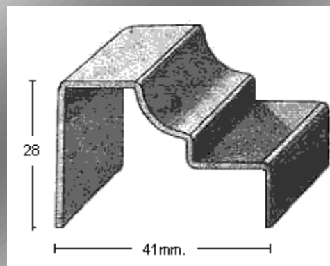
PERFIL 1813 (1mm.)
