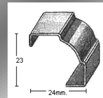
PERFIL 2031 (1mm.)
