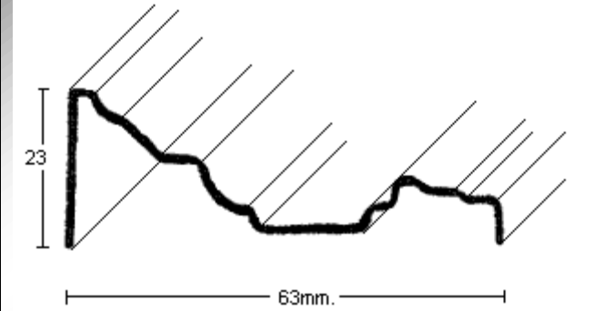
PERFIL 2770 (1,2mm.)
