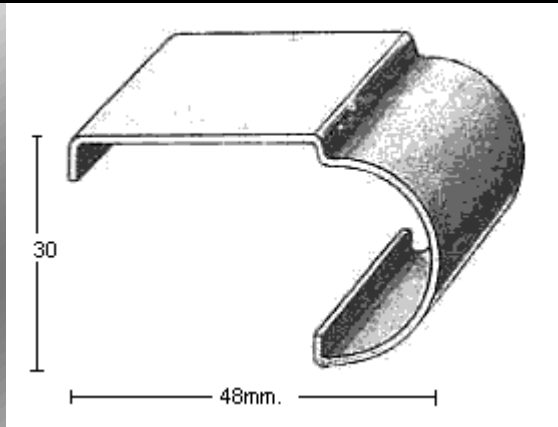
PERFIL 1915 (1,5mm.)
