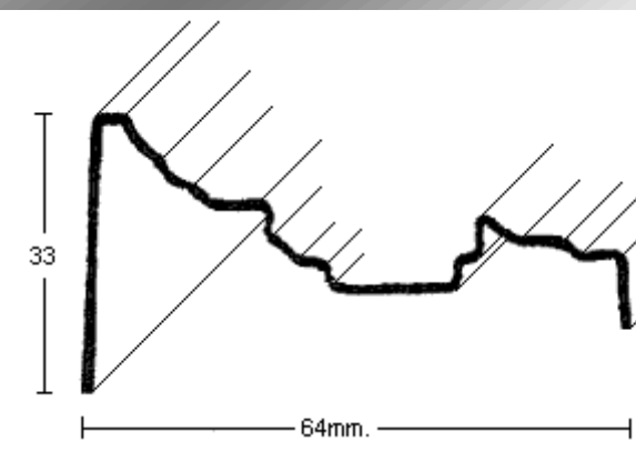
PERFIL 2548 (1,5mm.)
