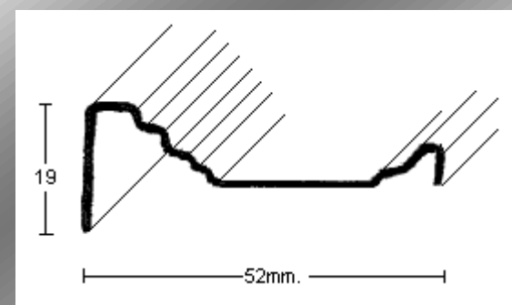
PERFIL 2770 (1,2mm.)
