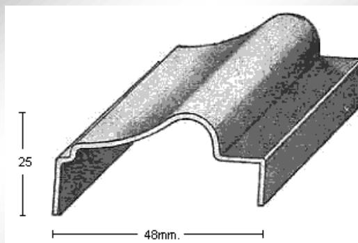
PERFIL 1813 (1mm.)
