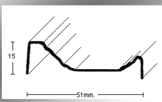
PERFIL 2769 (1,2mm.)
