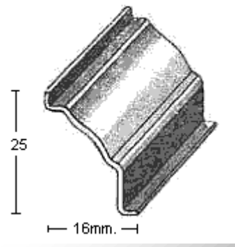
PERFIL 1850 (1mm.)
