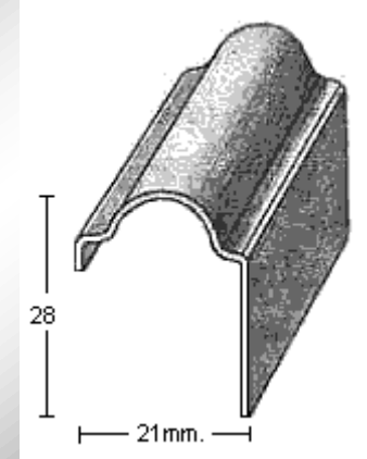
PERFIL 2031 (1mm.)
