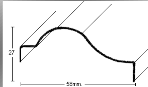
PERFIL 1947 (1mm.)
