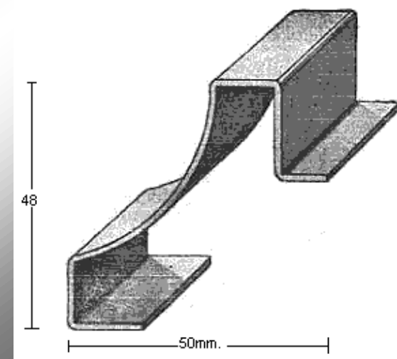
PERFIL 2014 (1,5mm.)
