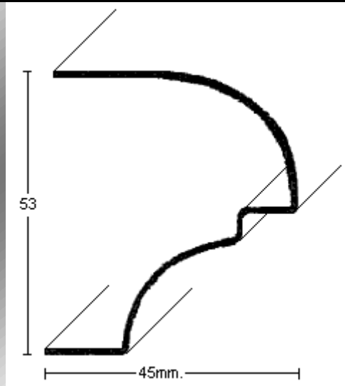
PERFIL 2662 (1,2mm.)
