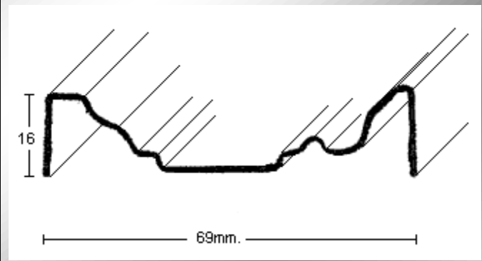
PERFIL 2663 (1,2mm.)
