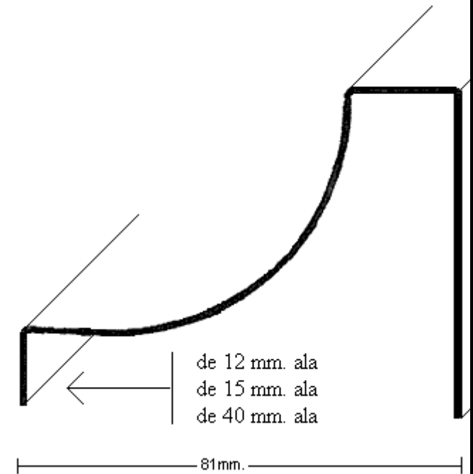
PERFIL 2663 (1,2mm.)
