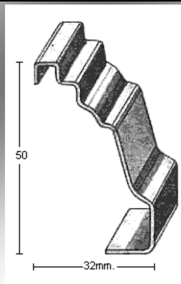
PERFIL 1876 (1mm.)
