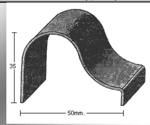
PERFIL 2774 (1,2mm.)
