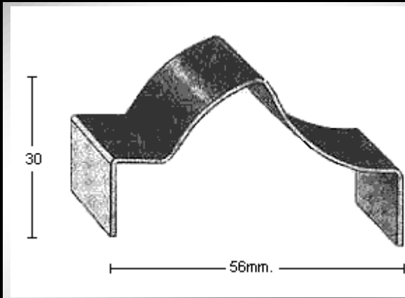
PERFIL 2102 (1mm.)
