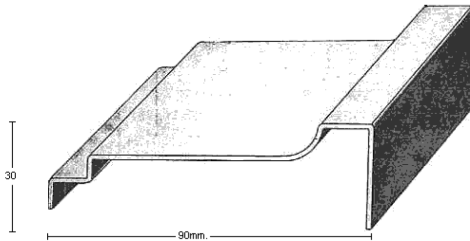
PERFIL 2267 (1,5mm.)
