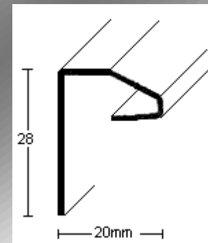
PERFIL 2606 (0,8mm.)
