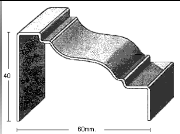
PERFIL 2228 (1,2mm.)
