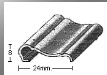
PERFIL 1901 (1mm.)
