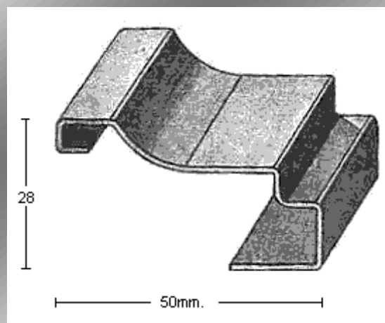
PERFIL 2102 (1mm.)
