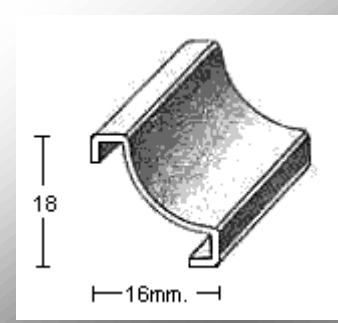
PERFIL 1918 (0,8mm.)
