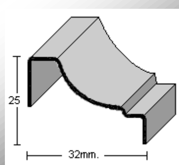
PERFIL 2776 (1mm.)
