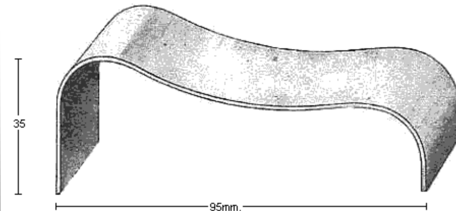
PERFIL 1878 (1,2mm.)
