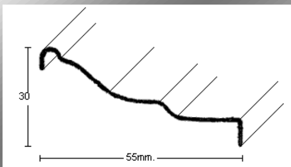
PERFIL 2772 (1,2mm.)
