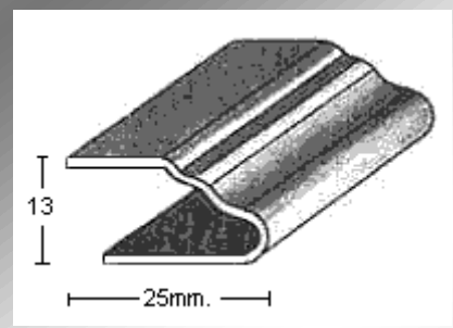
PERFIL 1918 (0,8mm.)
