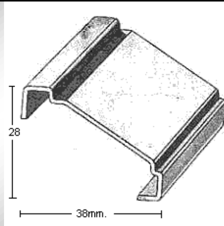
PERFIL 1876 (1mm.)
