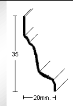
PERFIL 1781 (1mm.)
