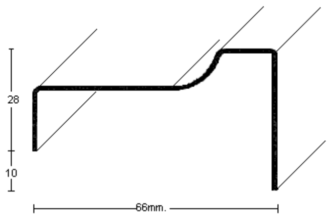
PERFIL 2603 (1,5mm.)
