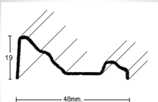
PERFIL 2769 (1,2mm.)
