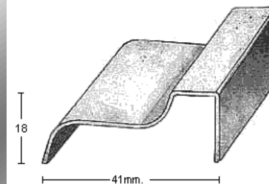
PERFIL 1879 (1mm.)
