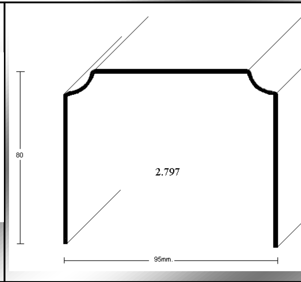
PERFIL 2797 (1,5mm.)
