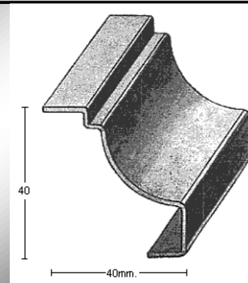
PERFIL 2025 (1mm.)
