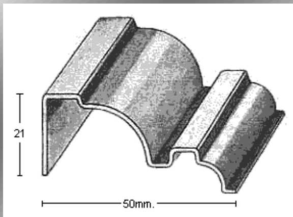
PERFIL 1900 (1mm.)
