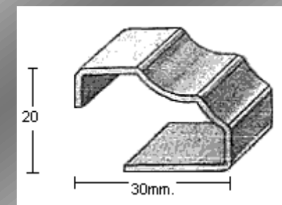
PERFIL 2004 (1mm.)
