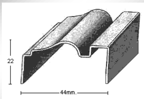
PERFIL 1828 (1,2mm.)
