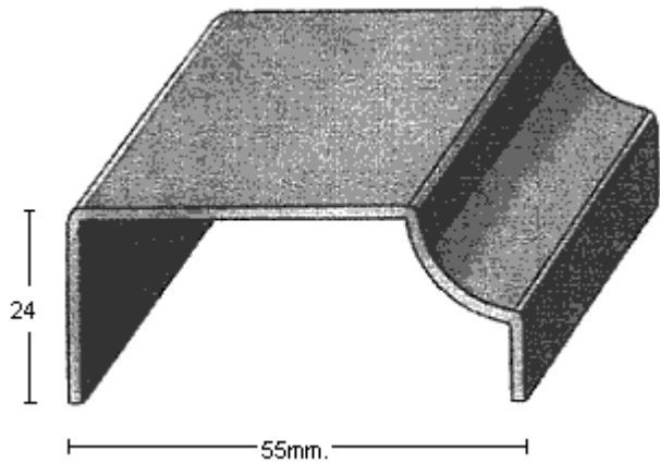
PERFIL 2191 (1mm.)
