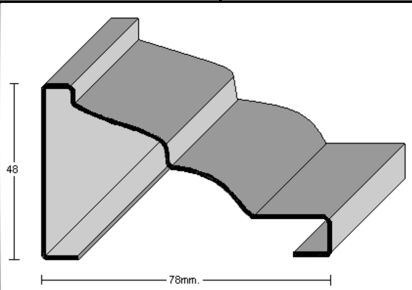
PERFIL 2720 (0,8mm.)
