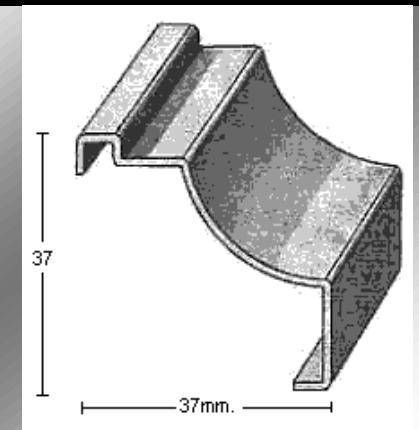
PERFIL 2747 (1mm.)
