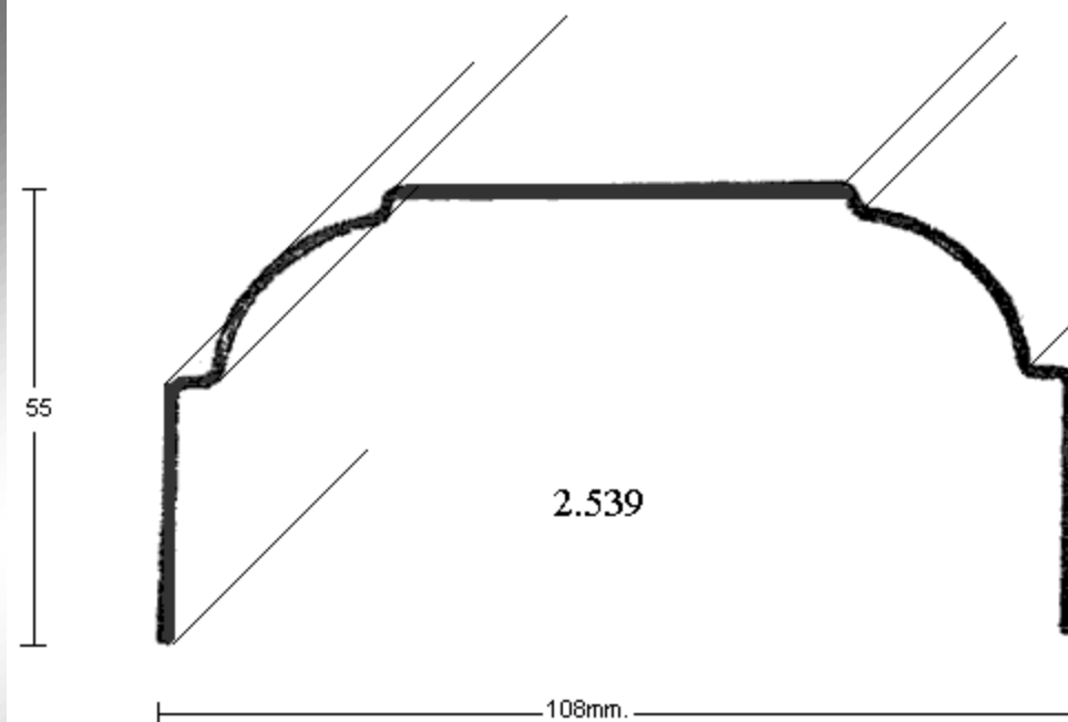
PERFIL 2539 (1,5mm.)
