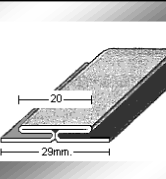
PERFIL 2309 (hueco 2mm.)
