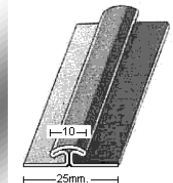
PERFIL 1557 (hueco 1,5mm.)
