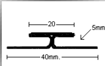
PERFIL 1780 (hueco 5mm.)
