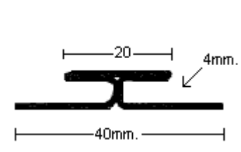
PERFIL 1780 (hueco 4mm.)
