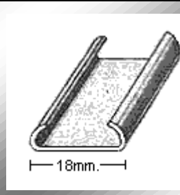
PERFIL 1217 (0,8mm.)
