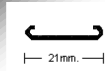
PERFIL 1772 (1,2mm.)
