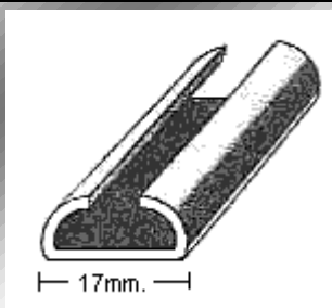
PERFIL 1108 (0,8mm.)
