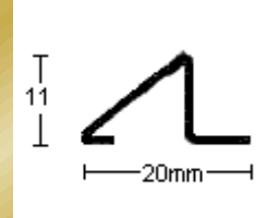
PERFIL 2544 (1mm.)
