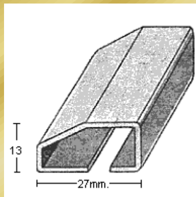
PERFIL 2353 (1,5mm.)
