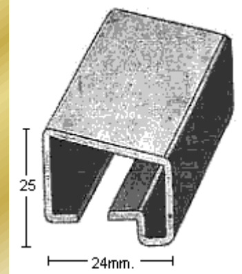
PERFIL 1829 (1,2mm.)
