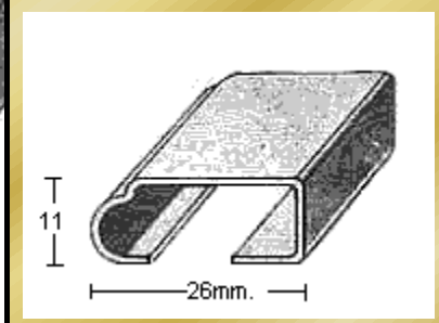
PERFIL 1897 (1mm.)
