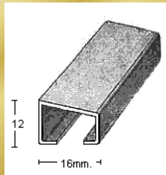
PERFIL 1830 (1mm.)
