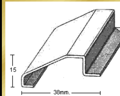
PERFIL 2063 (1,2mm.)
