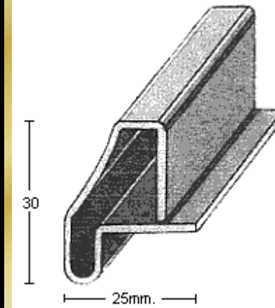
PERFIL 2372 (1,5mm.)
