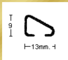
PERFIL 1734 (1mm.)
