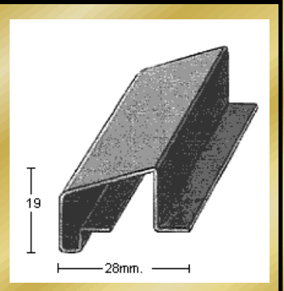
PERFIL 2450 (1,2mm.)
