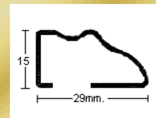
PERFIL 2727 (1,2mm.)
