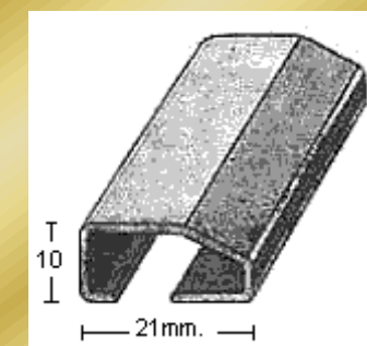
PERFIL 2030 (1,2mm.)
