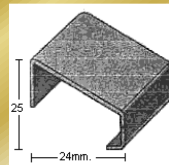
PERFIL 2198 (1,2mm.)
