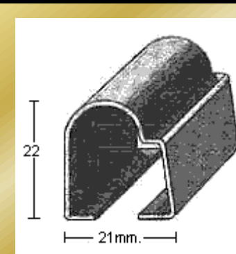
PERFIL 2157 (1mm.)
