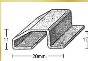
PERFIL 2251 (1,2mm.)
