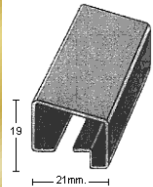
PERFIL 2451 (1,2mm.)
