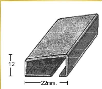
PERFIL 2323 (1mm.)
