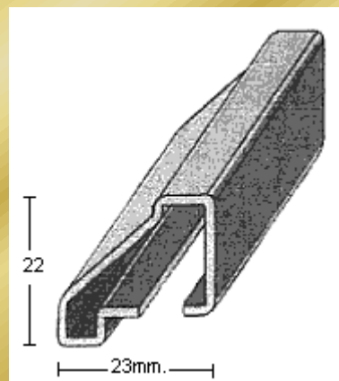
PERFIL 2367 (1,5mm.)
