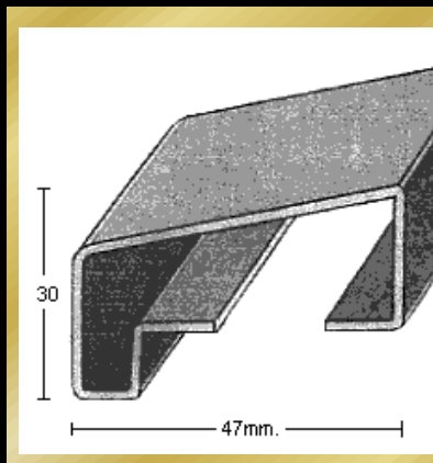
PERFIL 2452 (1,5mm.)
