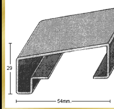
PERFIL 2456 (1,5mm.)
