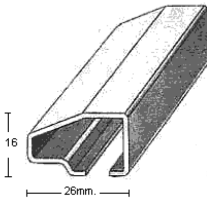
PERFIL 1867 (1,2mm.)
