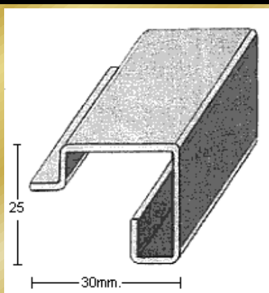
PERFIL 237 (1,5mm.)
