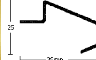
PERFIL 2592 (1,2mm.)
