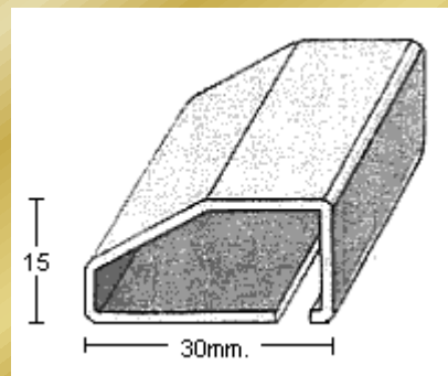
PERFIL 2408 (1,5mm.)
