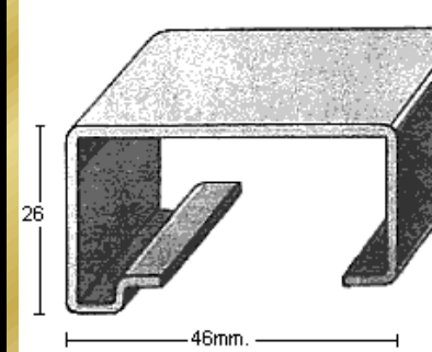
PERFIL 2342 (1,5mm.)
