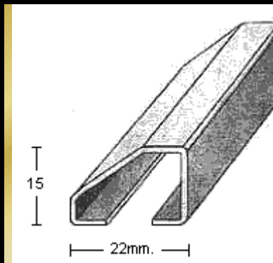
PERFIL 1889 (1,2mm.)
