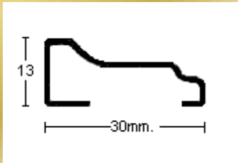
PERFIL 2738 (1mm.)
