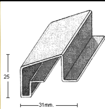
PERFIL 2426 (1,2mm.)
