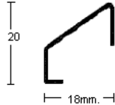
PERFIL 2519 (1mm.)
