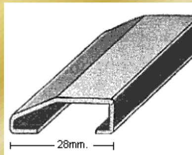
PERFIL 2300 (1,5mm.)
