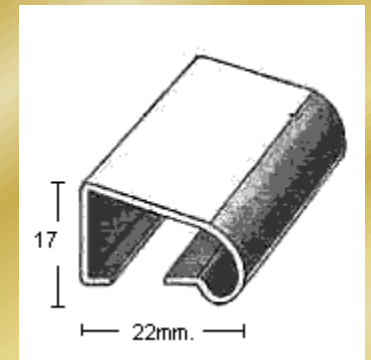
PERFIL 1838 (1mm.)
