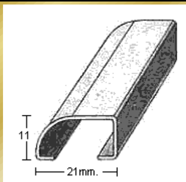
PERFIL 1914 (1mm.)
