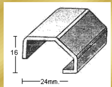
PERFIL 2224 (2mm.)
