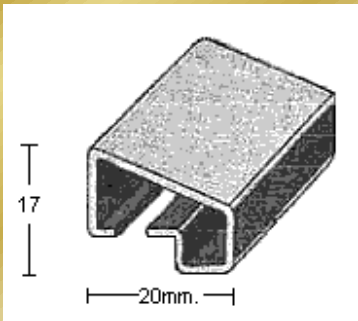
PERFIL 2264 (1,2mm.)
