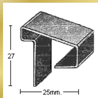
PERFIL 2134 (1mm.)
