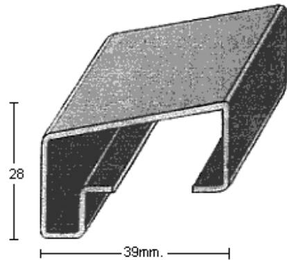
PERFIL 2453 (1,5mm.)
