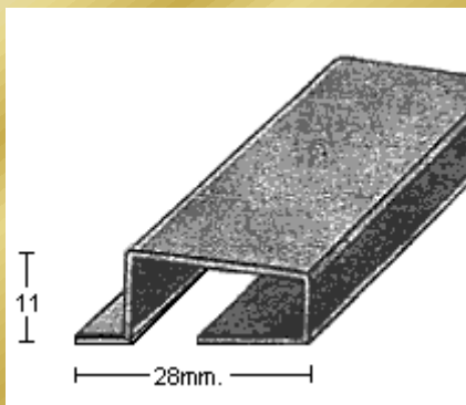
PERFIL 2324 (1mm.)
