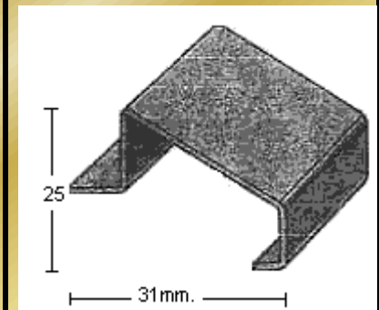
PERFIL 2199 (1,2mm.)
