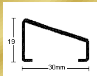
PERFIL 2629 (1,5mm.)
