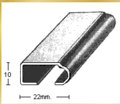
PERFIL 1807 (1mm.)
