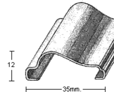
PERFIL 1947 (1mm.)
