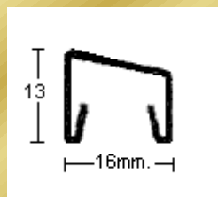
PERFIL 2610 (1mm.)
