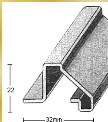
PERFIL 2368 (1,5mm.)
