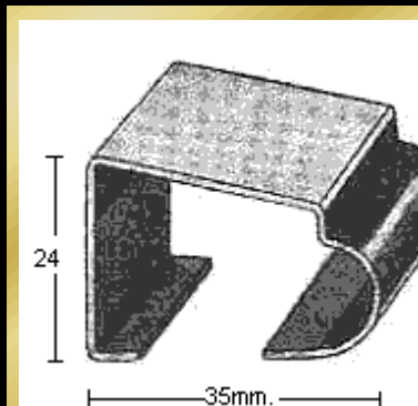
PERFIL 2156 (1mm.)
