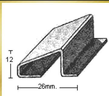
PERFIL 2119 (1mm.)
