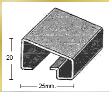
PERFIL 2271 (1,2mm.)
