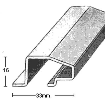
PERFIL 1868 (1,2mm.)
