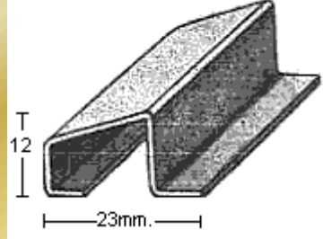
PERFIL 2177 (1mm.)
