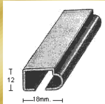
PERFIL 1815 (1mm.)
