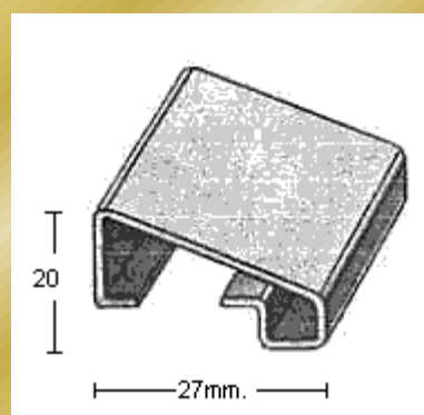
PERFIL 2053 (1mm.)
