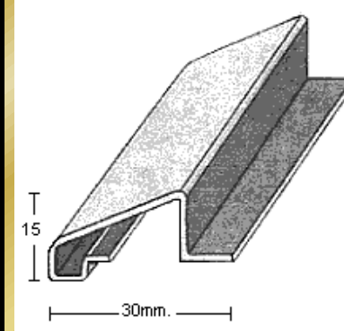
PERFIL 2462 (1mm.)
