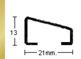
PERFIL 2569 (1mm.)
