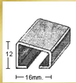
PERFIL 2179 (1,5mm.)
