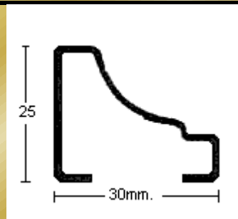
PERFIL 2618 (1,2mm.)
