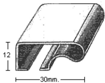
PERFIL 2045 (1,2mm.)
