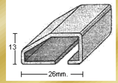
PERFIL 2222 (1 ó 1,5mm.)
