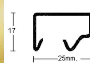
PERFIL 2694 (1,2mm.)
