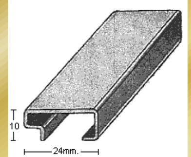
PERFIL 2360 (1,2mm.)
