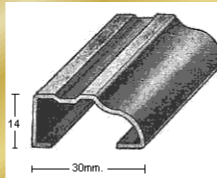
PERFIL 1812 (1,2mm.)
