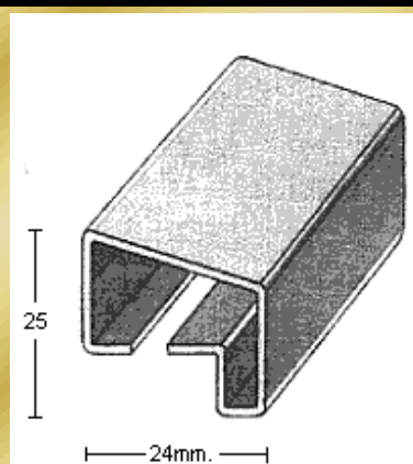
PERFIL 2427 (1,2mm.)
