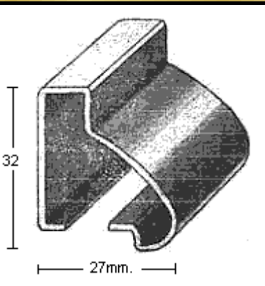
PERFIL 2187 (1,2mm.)
