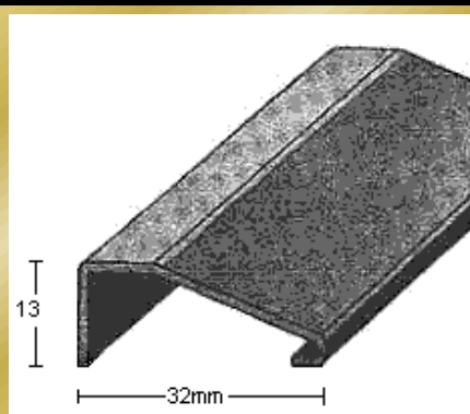
PERFIL 2145 (,5mm.)
