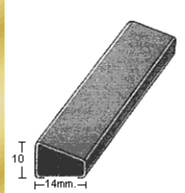
PERFIL 2448 (1mm.)
