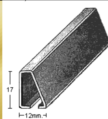
PERFIL 2358 (1,2mm.)
