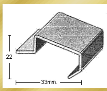
PERFIL 2272 (1,2mm.)
