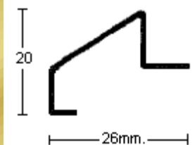
PERFIL 2518 (1mm.)
