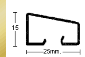
PERFIL 2609 (1mm.)
