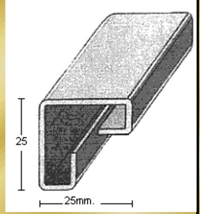
PERFIL 2370 (1,5mm.)
