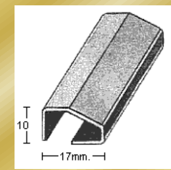
PERFIL 2392 (1mm.)
