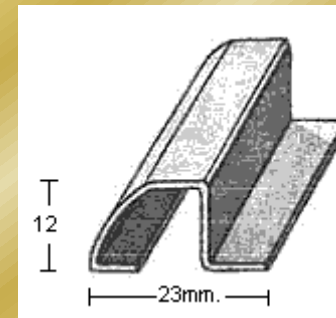
PERFIL 2054 (1mm.)
