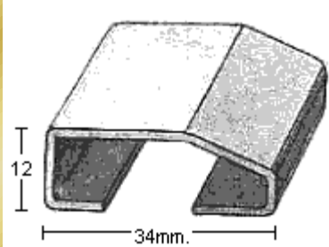
PERFIL 1944 (1mm.)
