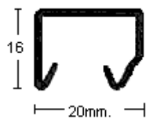
PERFIL 2697 (1,2mm.)
