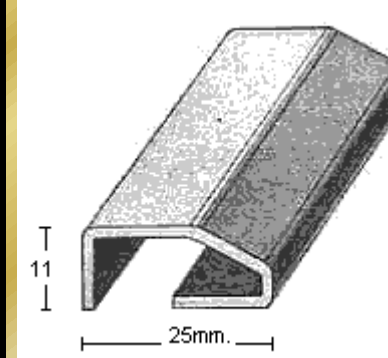
PERFIL 1816 (1,5mm.)
