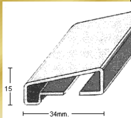
PERFIL 2369 (1,5mm.)
