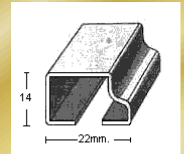
PERFIL 1820 (1mm.)
