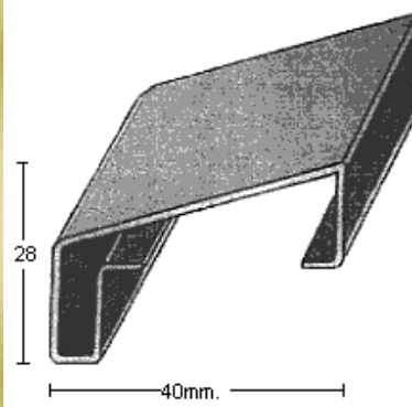
PERFIL 2454 (1,2mm.)
