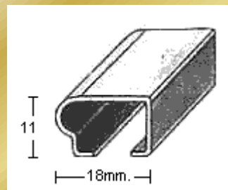
PERFIL 1919 (1mm.)
