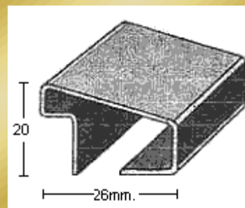
PERFIL 2135 (1mm.)
