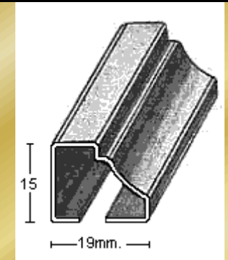
PERFIL 1928 (1mm.)
