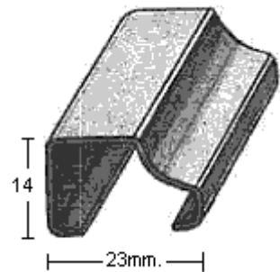
PERFIL 1931 (1mm.)
