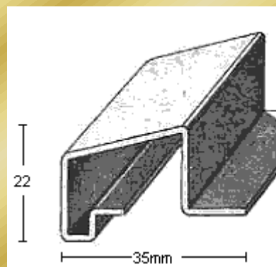
PERFIL 1837 (1,2mm.)
