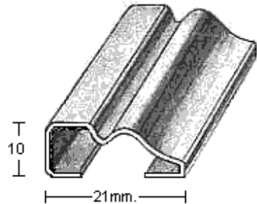
PERFIL 1941 (1mm.)
