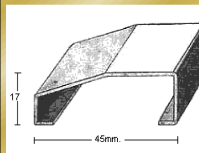
PERFIL 1842 (1,2mm.)
