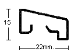
PERFIL 2718 (1mm.)
