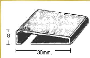
PERFIL 2169 (1,2mm.)
