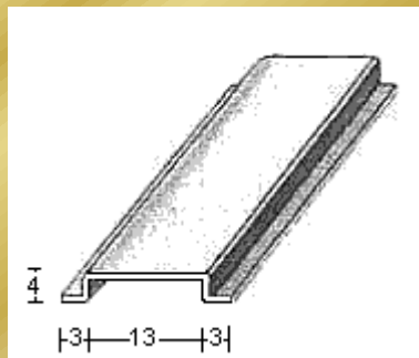
PERFIL 1494 (1mm.)
