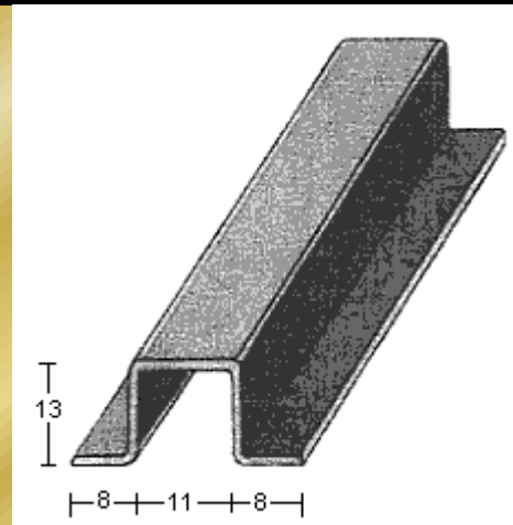
PERFIL 2380 (1,5mm.)
