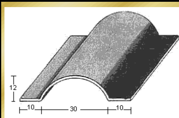
PERFIL 1615 (1,2mm.)
