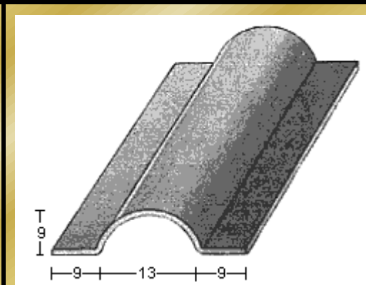
PERFIL 2437 (1,2mm.)
