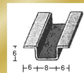
PERFIL 1374 (1mm.)
