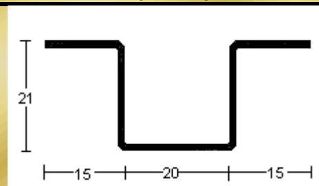
PERFIL 2729 (1,2mm.)
