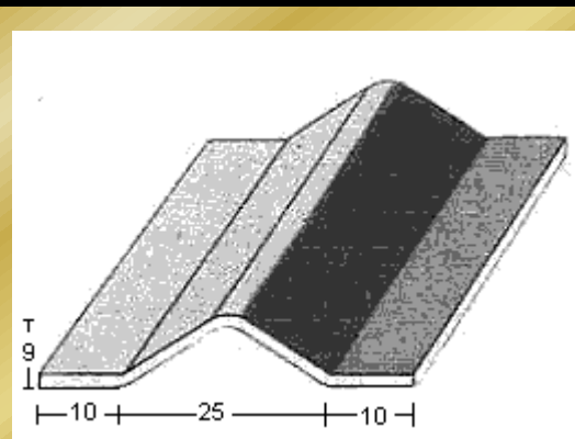
PERFIL 1587 (1,5mm.)
