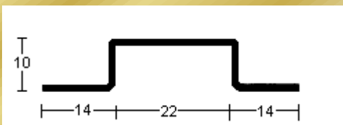
PERFIL 2709 (1,5mm.)
