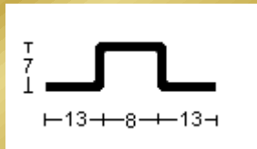
PERFIL 1744 (0,8mm.)
