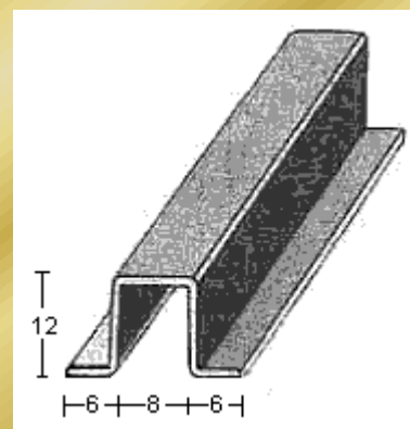
PERFIL 1518 (1mm.)
