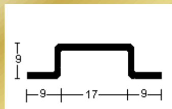
PERFIL 2734 (1,5mm.)
