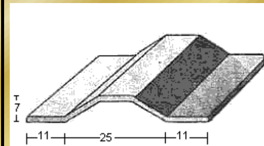
PERFIL 1366 (1,5mm.)
