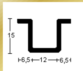
PERFIL 1777 (1,5mm.)
