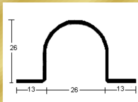
PERFIL 2725 (1,5mm.)
