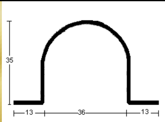
PERFIL 2746 (1,5mm.)
