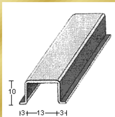
PERFIL 2374 (1mm.)
