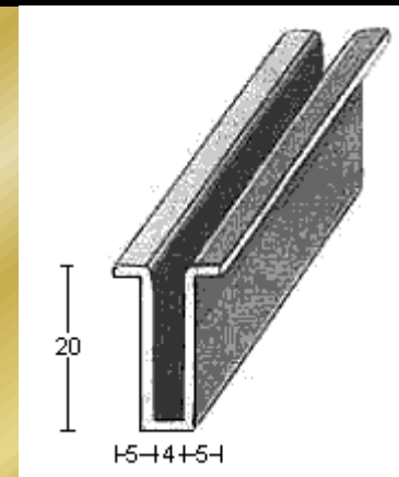
PERFIL 1578 (1,5mm.)
