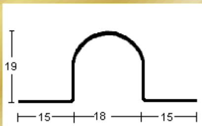
PERFIL 1790 (1mm.)
