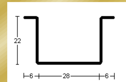
PERFIL 2676 (1,2mm.)
